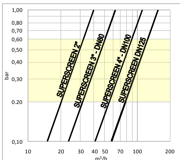
PERDITE DI CARICO IN ZONA DI LAVORO SERIE SUPERSCREEN (FLOW RESISTANCE IN WORK AREA SUPERSCREEN SERIES)
